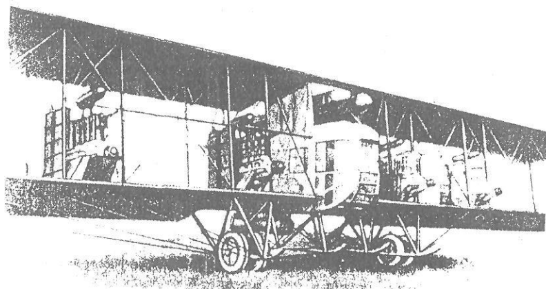
Русский военный 4-х моторный самолёт "Илья Муромец". Экипаж 8 человек. Поднимал до 800 кг бомб. К началу войны было построено 22 самолёта, а всего 73.
